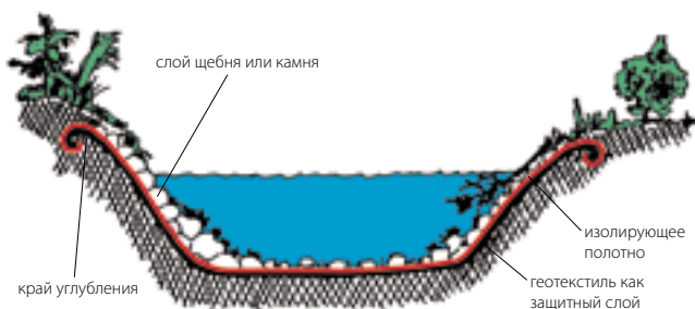
Схема пруда, изолированного материалом фирмы Schedetal
